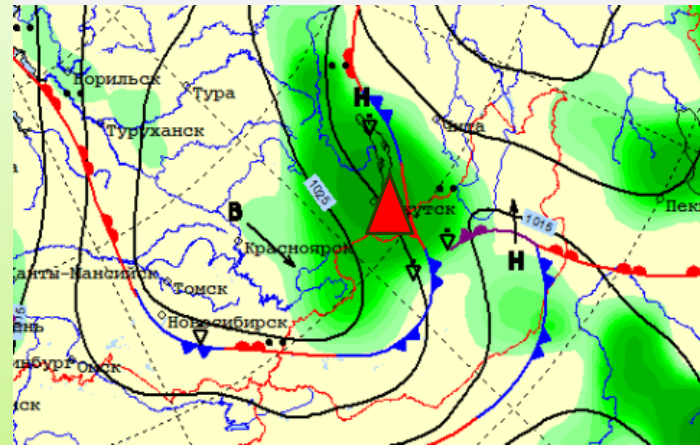
Приземное давление и атмосферные фронты
