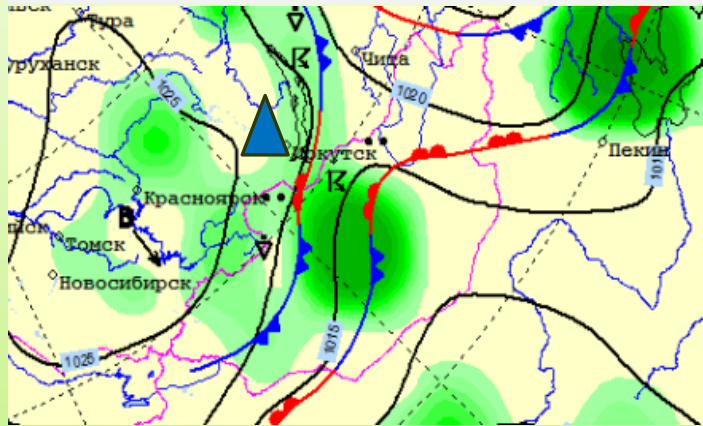
Приземное давление и атмосферные фронты
