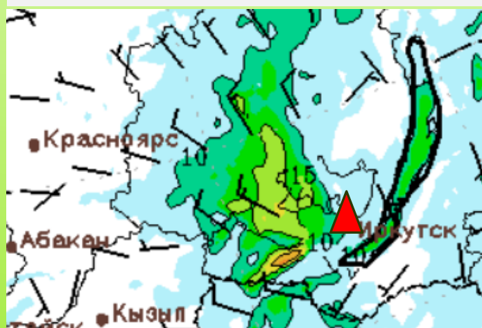
Ветер у поверхности Земли
