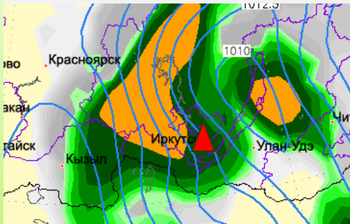
Приземное давление и атмосферные осадки
