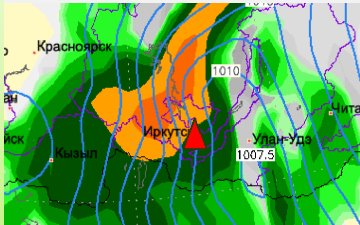
Приземное давление и атмосферные осадки
