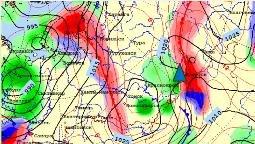
Приземное давление и атмосферные фронты
