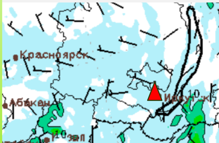
Ветер у поверхности Земли
