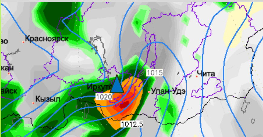
Приземное давление и атмосферные осадки
